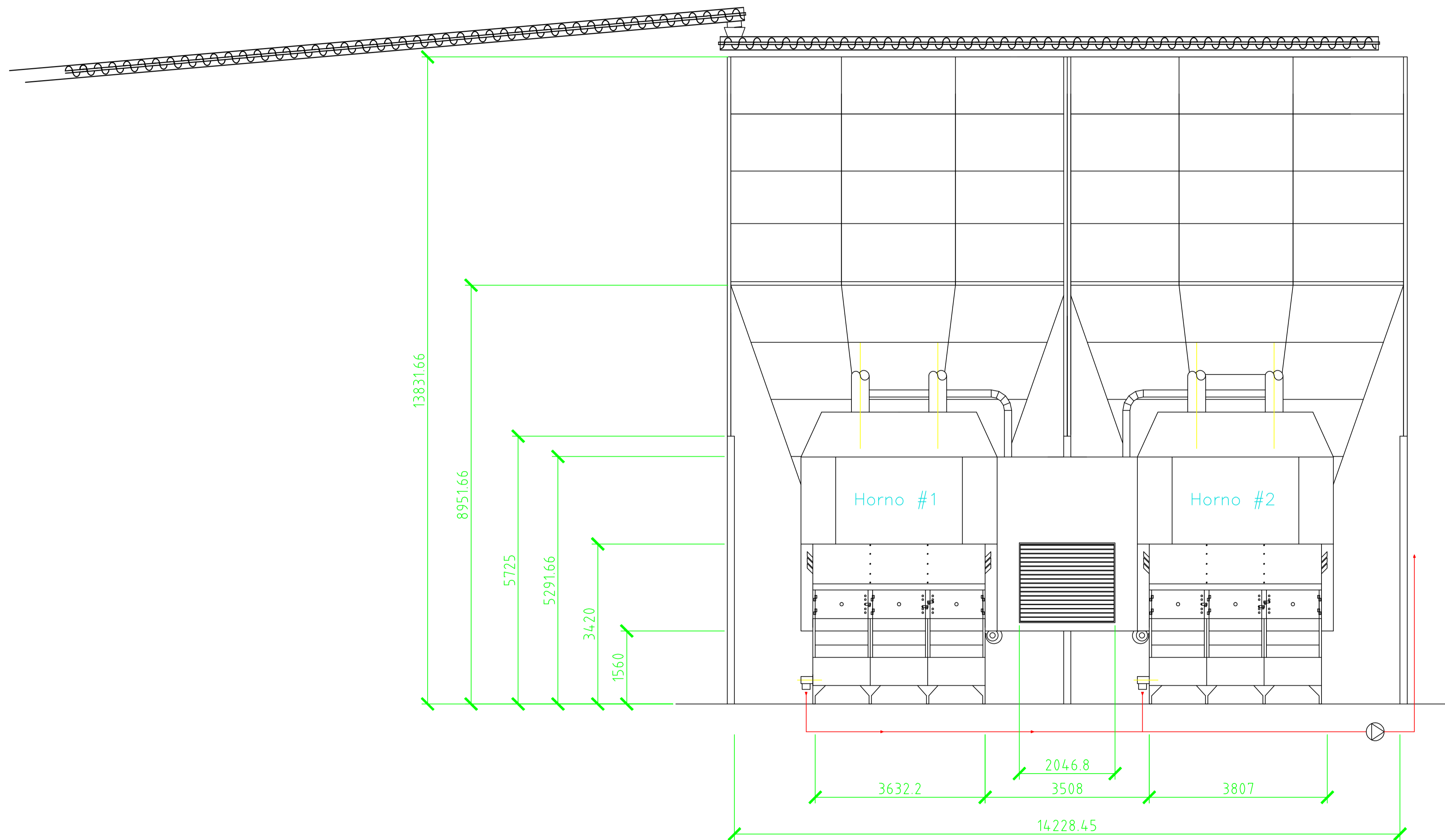
Vista A-A
